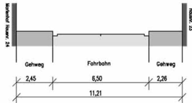
Straßenquerschnitt B 8 Marienhof
