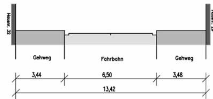
Straßenquerschnitt B 8 Schwanengasse
